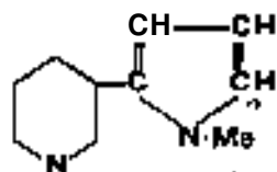
Nicotyzins, 0-004.
