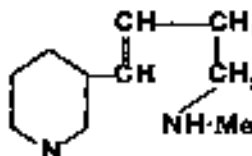
Metanicoline, 0-005.
